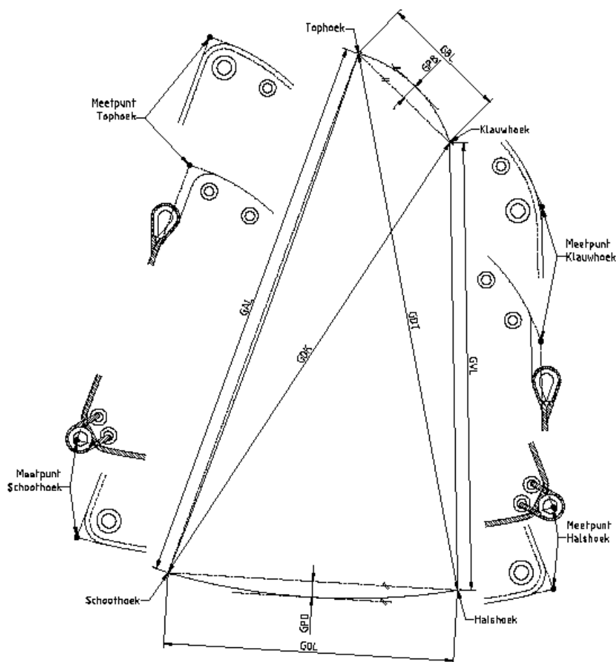
Maatvoering Grootzeil
